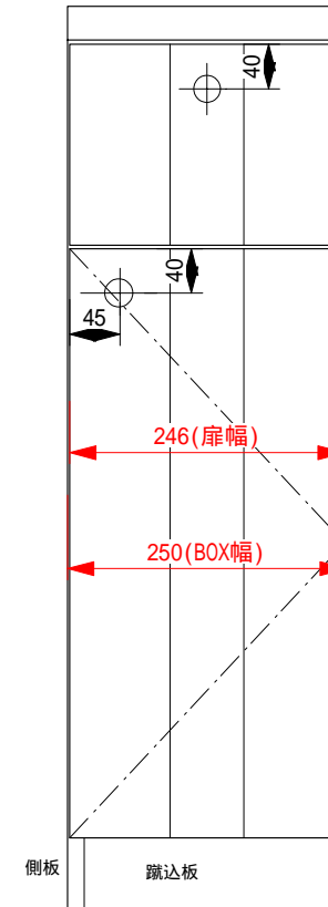
引出板、扉断面
