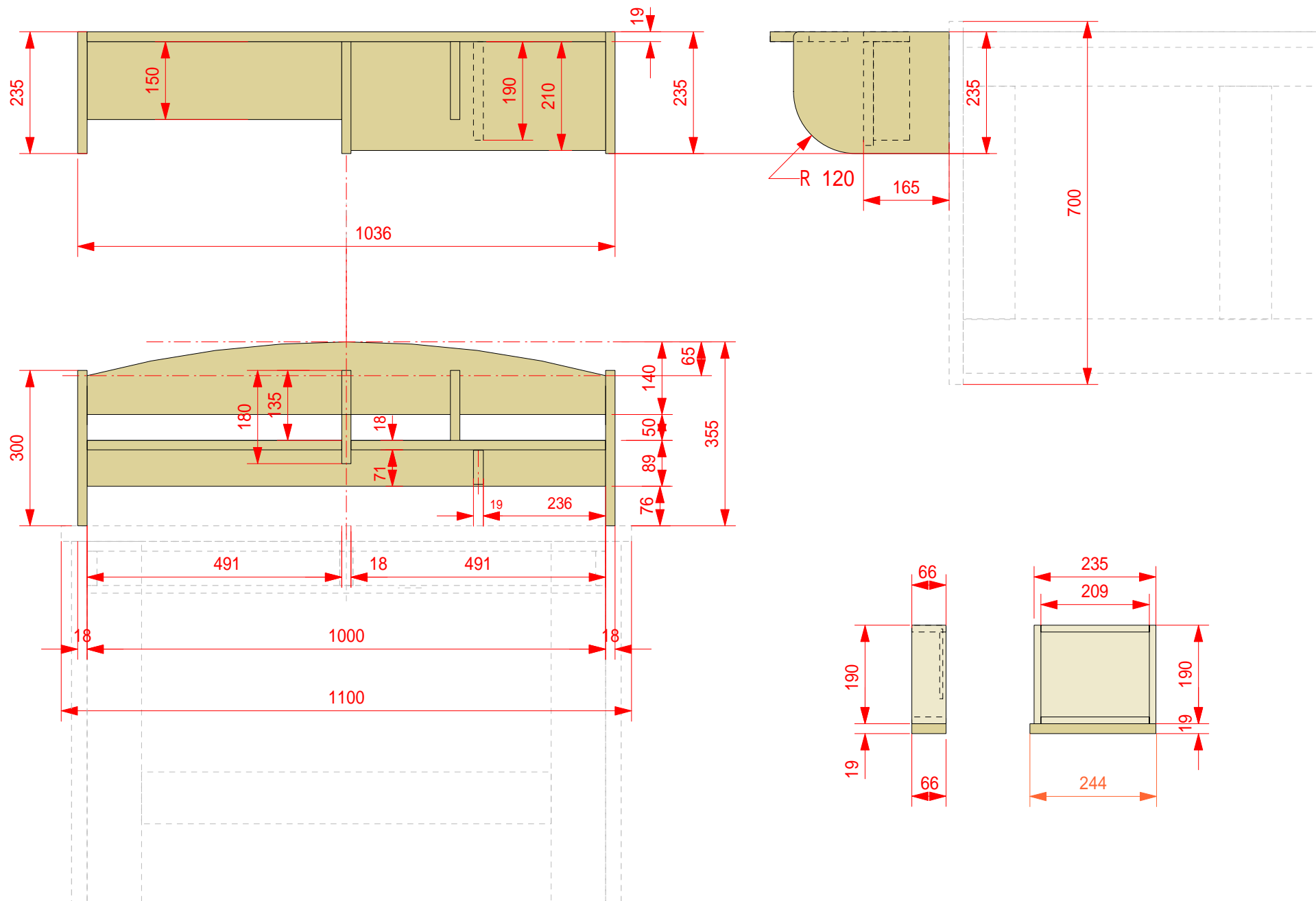
学習机 (本棚)
